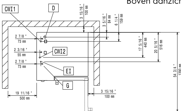
Boven aanzicht
